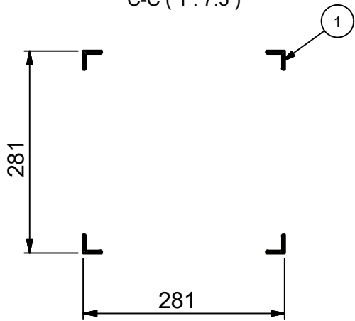
C-C ( 1 : 7.5 )
