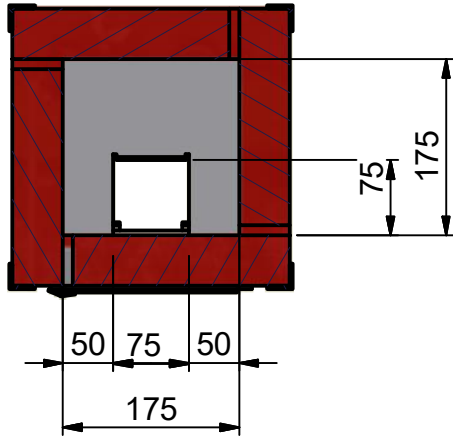
A-A ( 1 : 7.5 )
