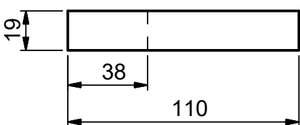
DESARROLLO PROPUESTO ( 1 : 2.5 )
