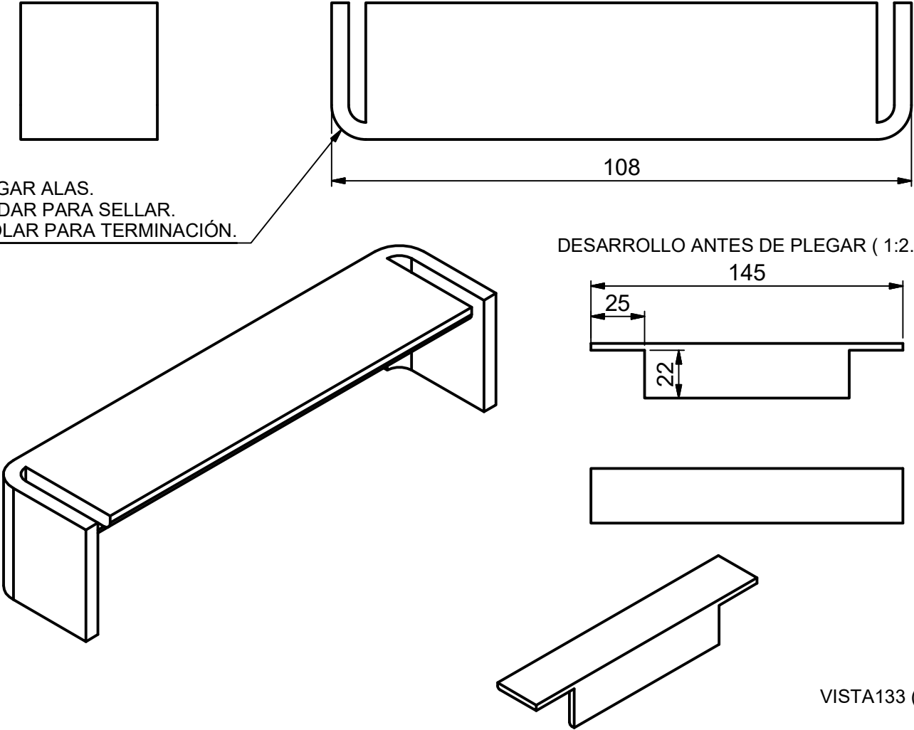
POS4 ( 1:1 )
