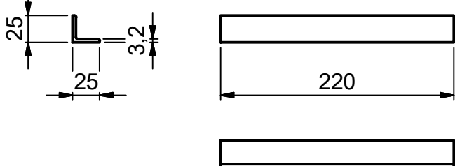
POS2 ( 1 : 5 )
