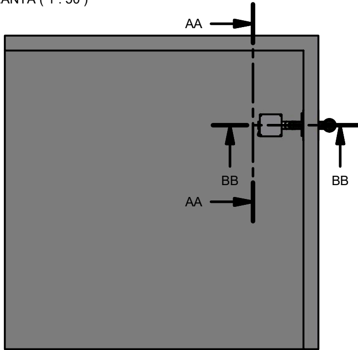
PLANTA ( 1 : 50 )
