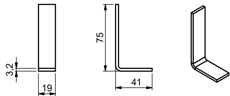
POS1 ( 1 : 2.5 )
