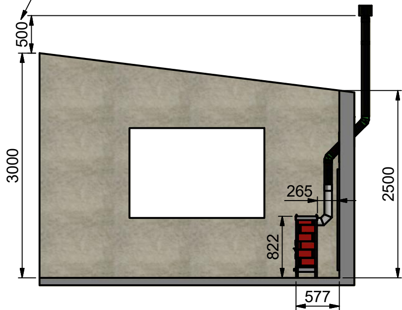
VISTA153 ( 1 : 50 )
