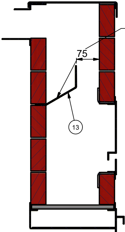
POS13 ( 1 : 5 )
