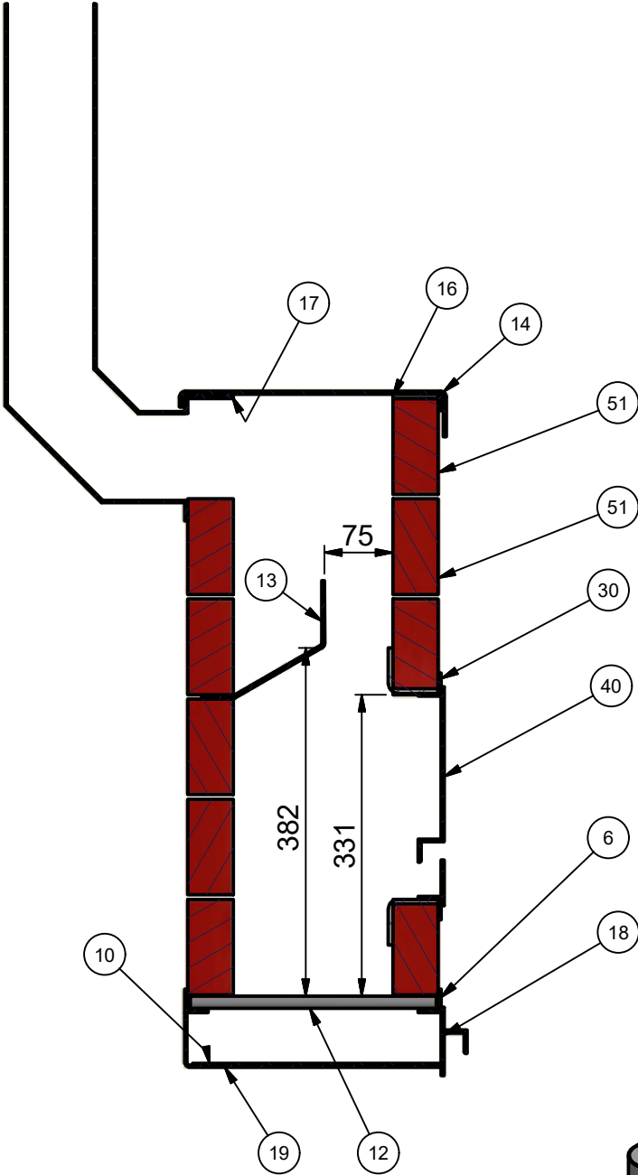
B-B ( 1 : 7.5 )
