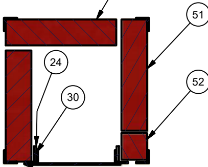
3-3 ( 1 : 7.5 )
