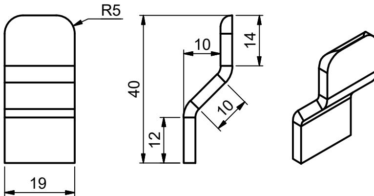
POS3 ( 1:1 )
