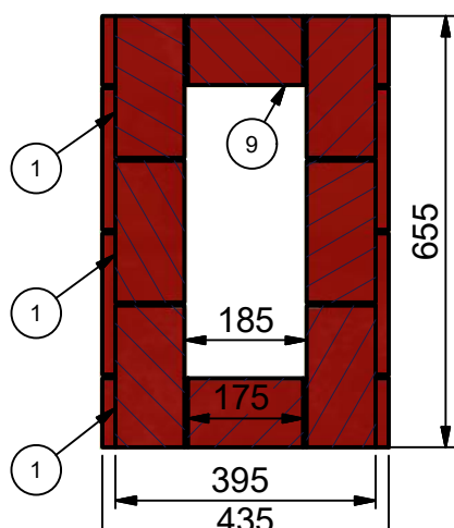
20-20 ( 1:12.5 ) (SE VE TAMBIÉN HILADA 19)
