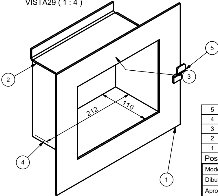
VISTA29 ( 1 : 4 )
