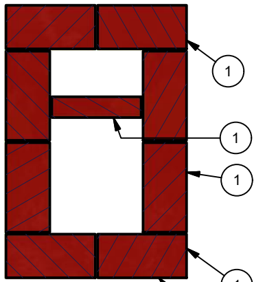
15-15 ( 1:12.5 )
